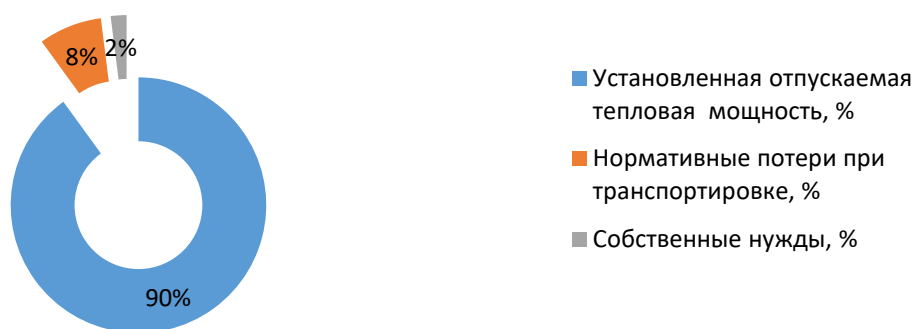
Распределение общего объема располагаемой тепловой энергии при нормативных потерях с.Колчаново, мкр-н "Алексино"
