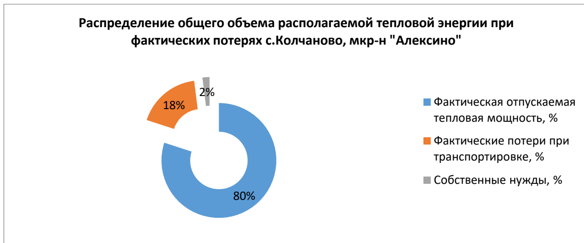
Диаграмма 1.2. Распределение общего объема располагаемой тепловой энергии (при фактических значениях потерь).
